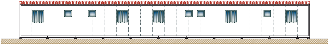
Alçado Lateral Esquerdo
