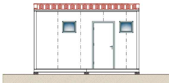
Alçado Principal
