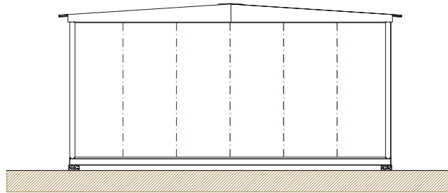
Alçado Lateral Esquerdo
