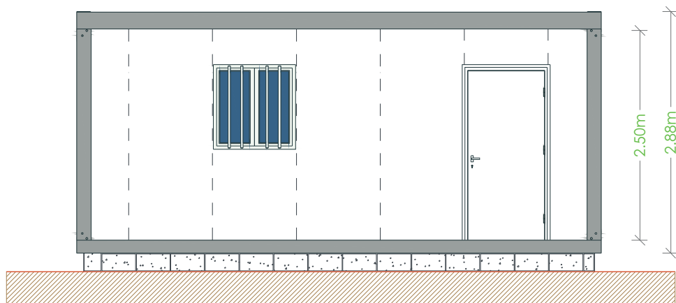
Alzado Frontal
