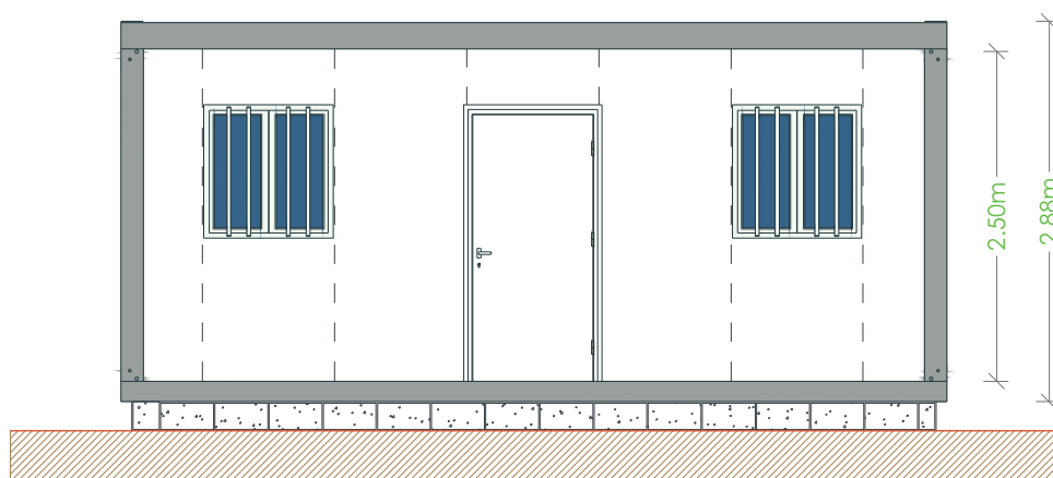
Alzado Frontal
