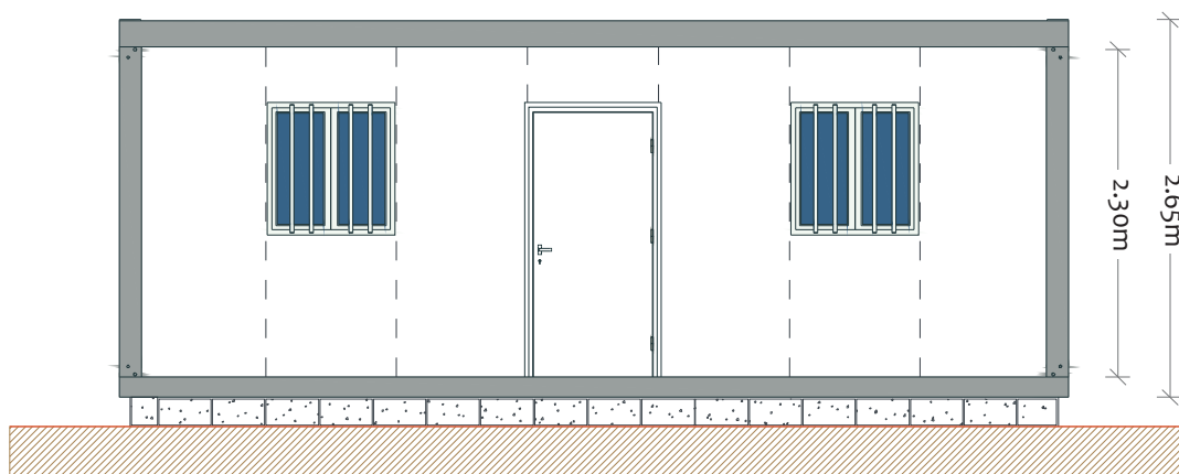
Alzado Frontal
